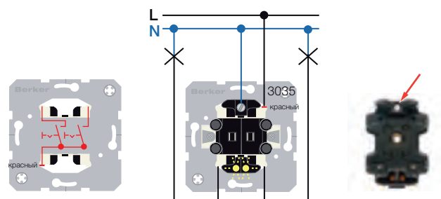
Рис 6: Двойной контрольный выключатель (элемент подсветки горит для каждой серии в положении «Вкл.»), клемма N (см. рис. справа)
