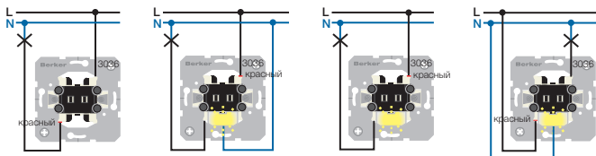
Рис 3: Выключатель/контрольный выключатель*: элемент подсветки горит в положении «Вкл.» / выключатель с подсветкой: элемент подсветки горит в положении «Выкл.» / выключатель с постоянной подсветкой*
