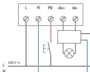
Рис 1: Подсоединение инфракрасного датчика присутствия DALI
