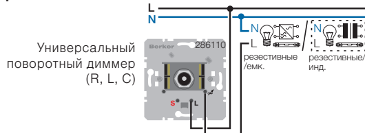
Рис 1: Выключение
