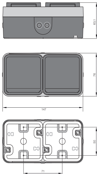
Рис 3: Розетка SCHUKO, 2-местная с откидной крышкой Розетка
