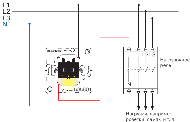
Рис 1: Кнопочный выключатель, переключающий контакт для гостиничной карты: элемент подсветки горит только в том случае, если гостиничная карта не вставлена.
