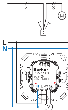
Рис 1: Одноичное управление
