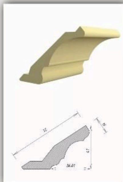
Карніз №2
