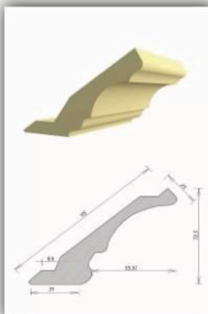
Карніз №1
