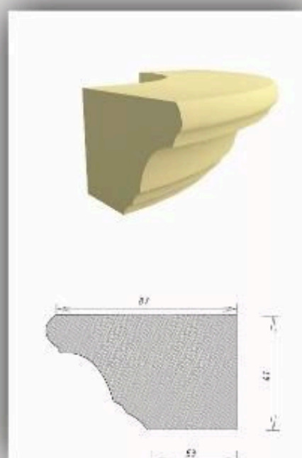
Карніз радіус №2
