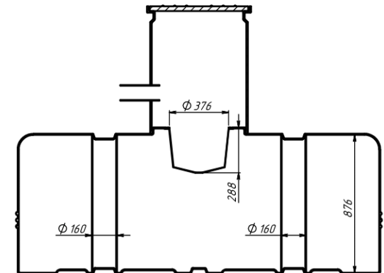
CROSS-SECTION A:A SCALE 1:12
