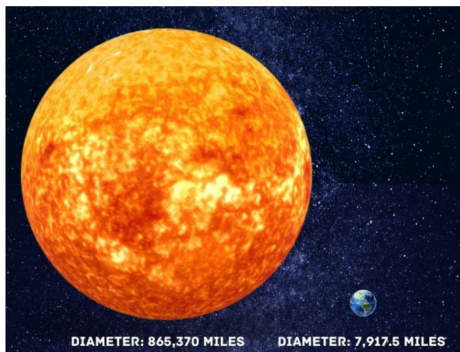
Сравнение Солнца и Земли
