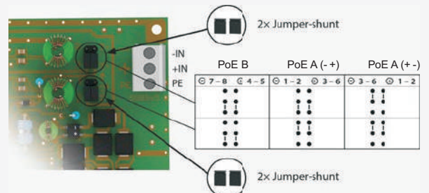
Мал. 5 Опис налаштувань режимів POE для DL-1G-POE-PCB-INJECTOR та DL-1G-POE-INJECTOR
