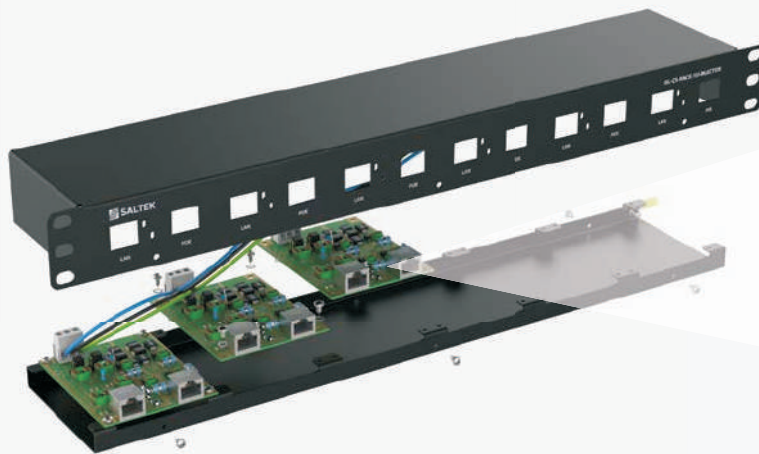
Мал. 4 DL-CS-RACK-1U-INJECTOR та встановлення модулів ПЗІП
