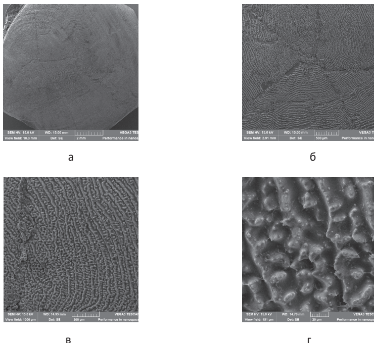
Рис. 3. Зображення фрагмента луски Товстолобика білого ( Hypophthalmichthys molitrix ): а) збільшено до 20 х ; б) збільшено до 70 х ; в) збільшено до 200 х ; г) збільшено до 1400 х
