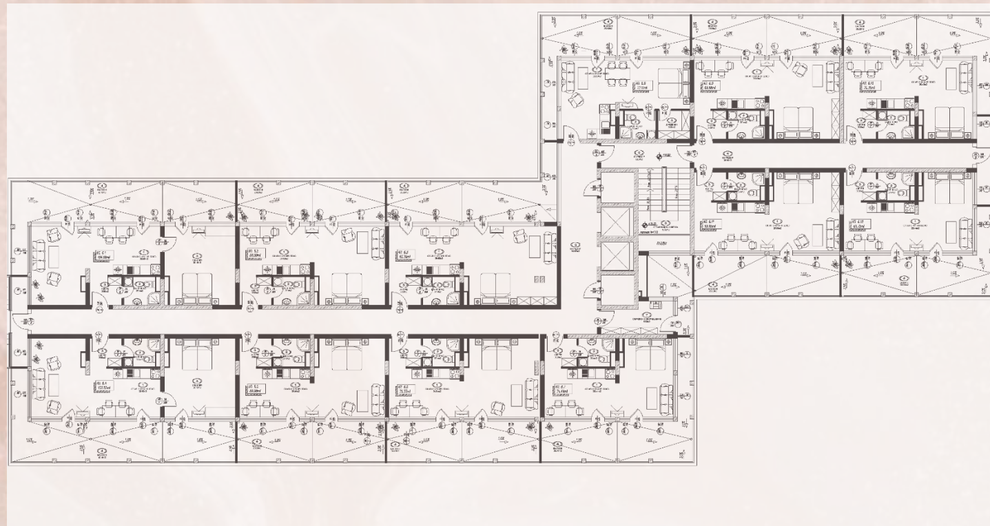
Разпределение на 6-ти етаж
