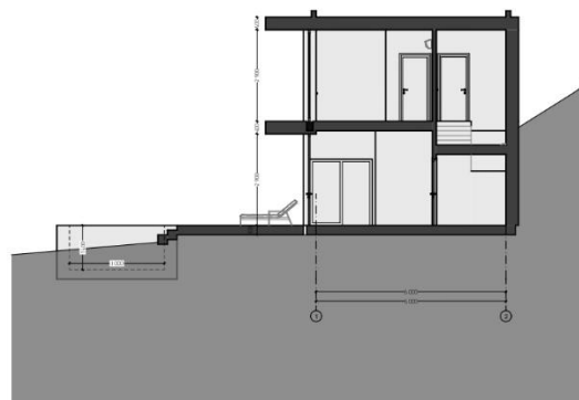
Условный разрез
