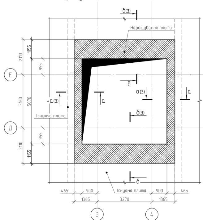
Схема дорощування монолітної плити
