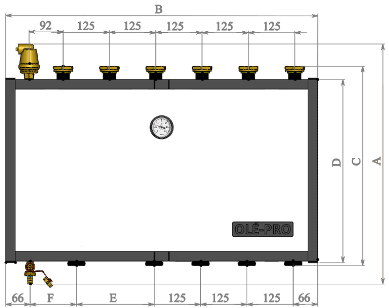
2. OTU-x-3-D-i
