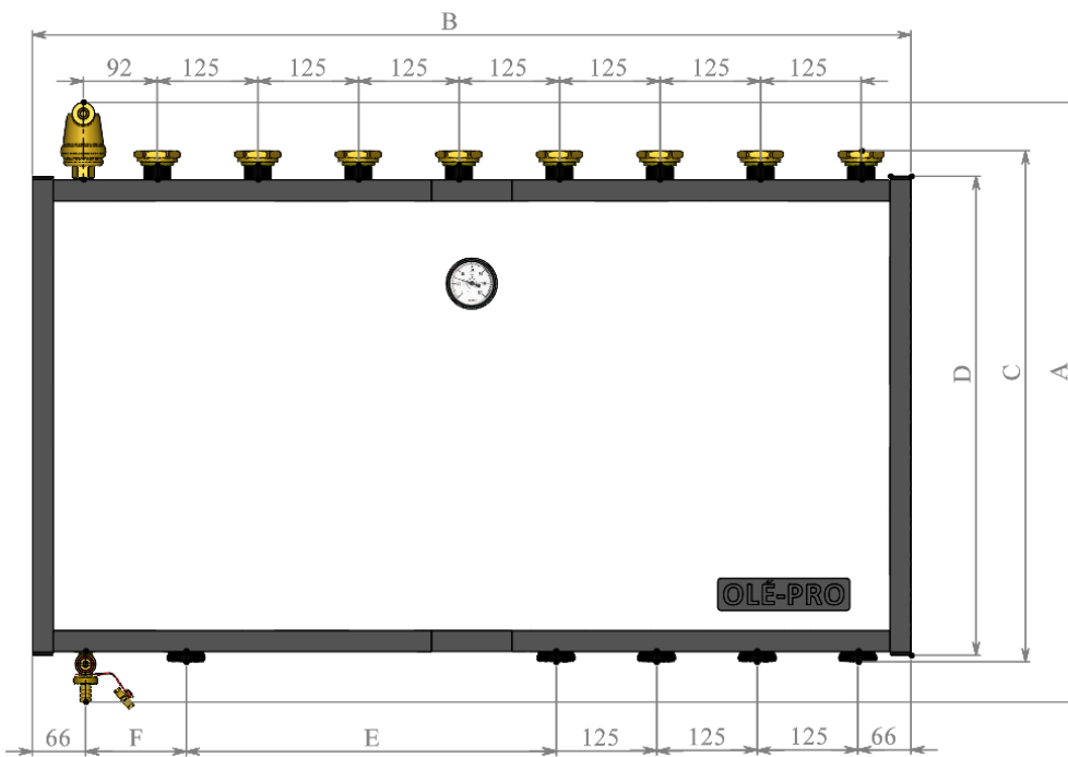
2. OTU-x-4-D-i
