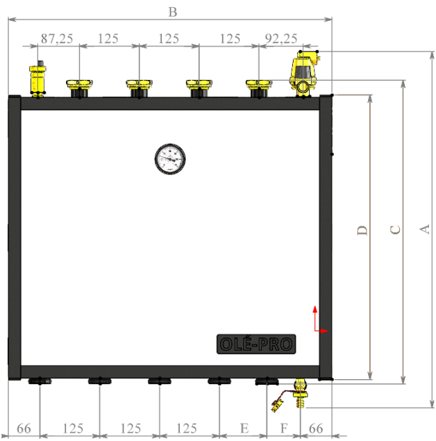
1. OTU-x-2-D-i
