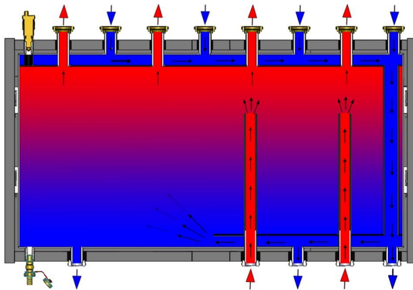
3. OTU-x-4-D-i
