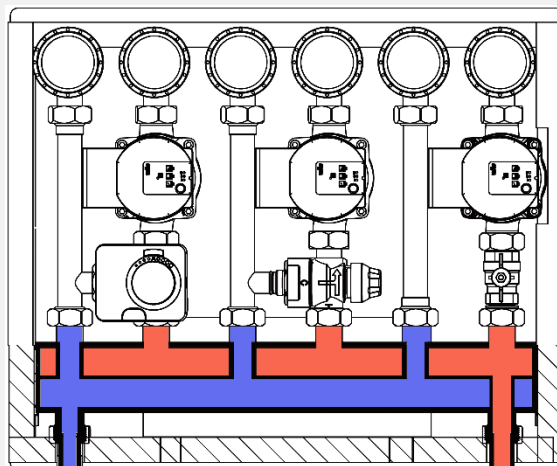
Схема руху теплоносія в OZB-A-35-3
