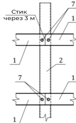
1-1 стиковий вузол
