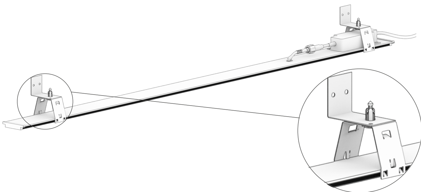
Кріплення - 4 Г - образне (для фасадів)
