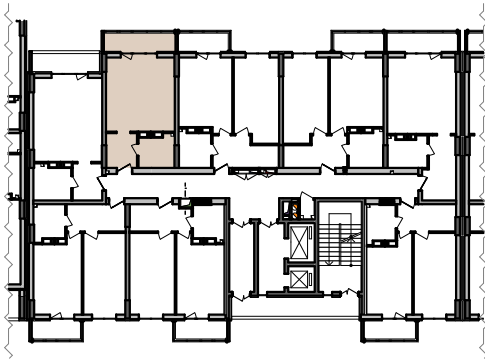
Схема розташування квартири на 6-8-ому поверсі
