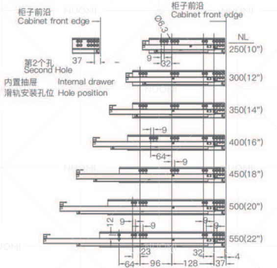
滑轨安装孔位 Hole position
