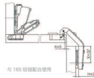
Hole Size 钻孔尺寸
