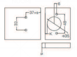
Hole Size 钻孔尺寸
