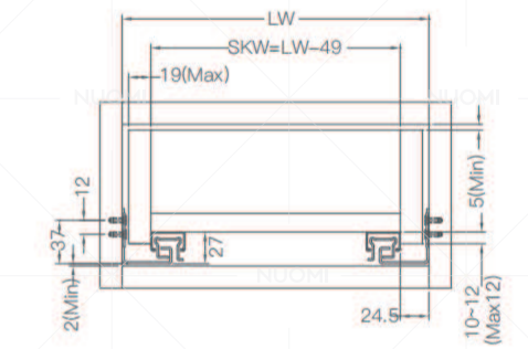
滑轨安装孔位 Hole position
