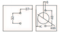
Hole Size 钻孔尺寸
