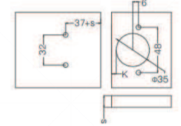
Hole Size 钻孔尺寸
