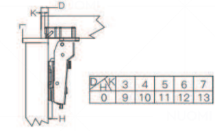
Half Overlay 中弯
