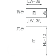
2. 用于 16/18mm 密度板的 裁切尺寸 Cutting dim.for 16/18mm chipboard
