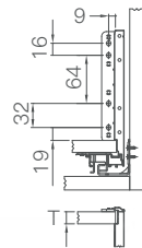
背板安装尺寸 Back installation dimensions 单位 unit:mm
