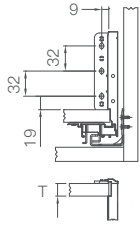
背板安装尺寸 Back installation dimensions 单位 unit:mm
