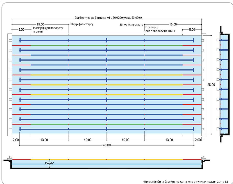
Схема 1. Басейн 50 м 8 доріжок
