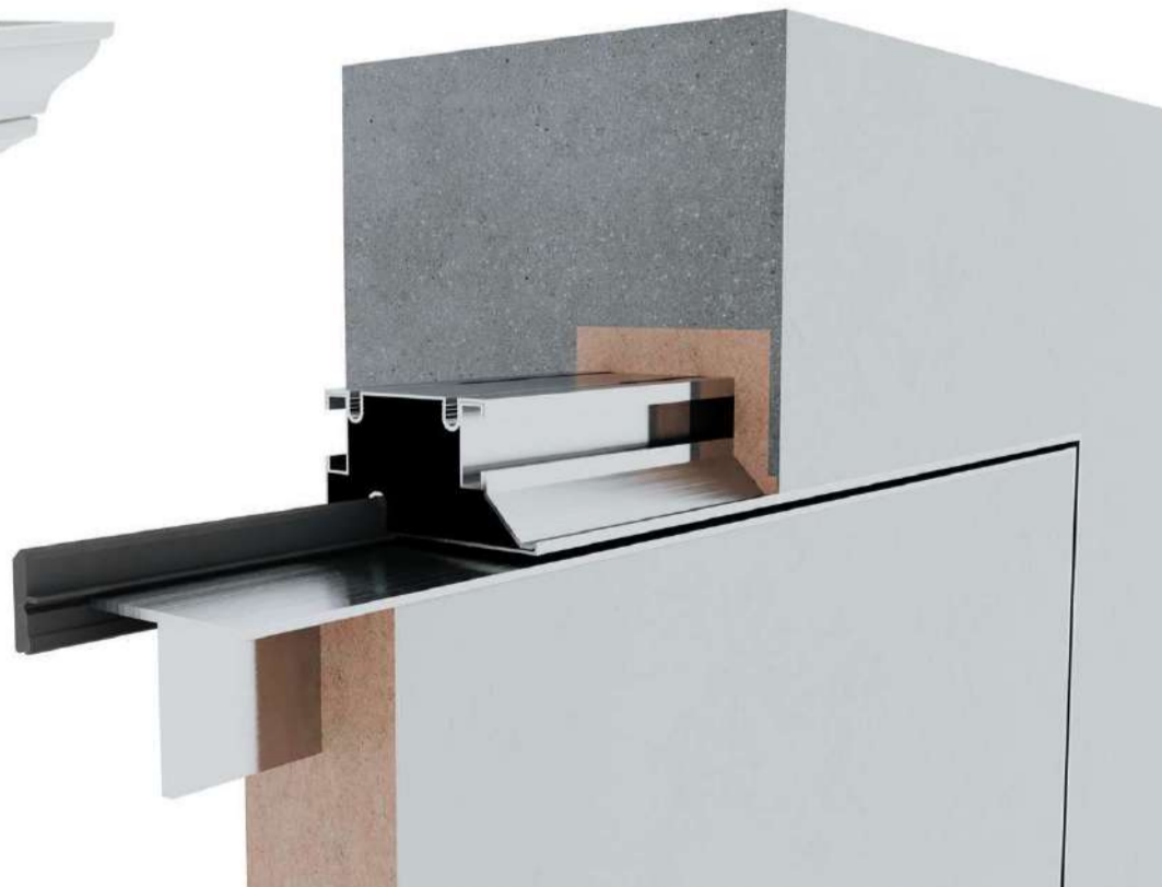
Прихований монтаж
