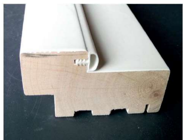
Коробка компонарна
