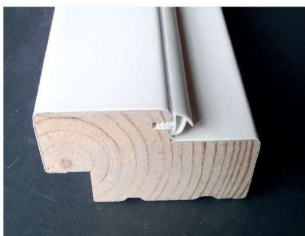
Коробка 31/36/45
