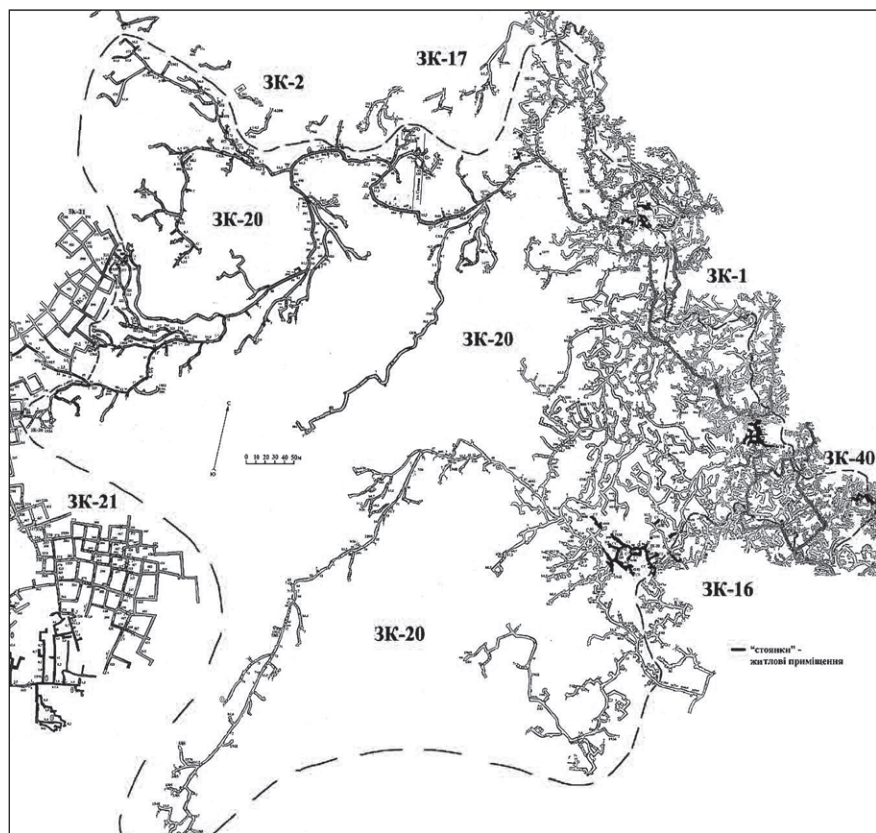
Мал.2. Схема катакомб району ЗК-20; Гідромет.
