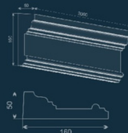
Карниз GE-17
