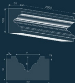
Рустова смуга LB-1
