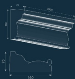
Карниз GE-10
