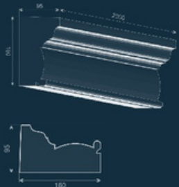
Карниз GE-10B
