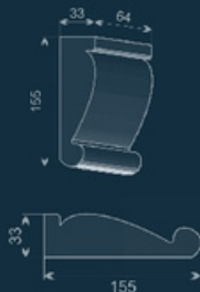
Кронштейн WE-1
