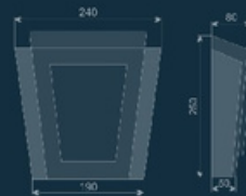
Замковий камінь ZE-3A
