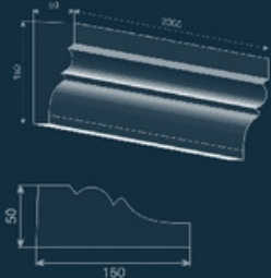
Карниз GE-23A
