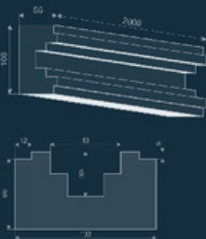
Рустова смуга LB-3
