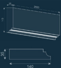
Молдинг LE-23
