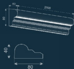
Молдинг LE-21
