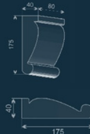
Кронштейн WE-2
