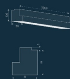
Рустова смуга LB-2A
