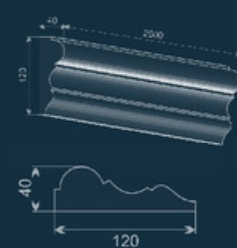
Молдинг LE-31A
