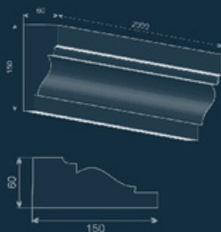
Карниз GE-22
