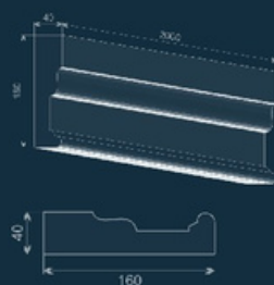
Карниз GE-16A
