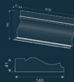
Молдинг LE-20
