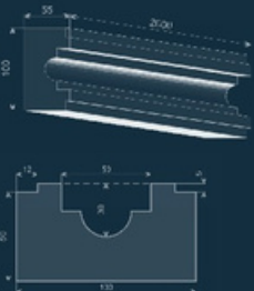
Рустова смуга LB-4
