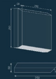
Босаж BE-2A
