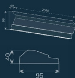
Молдинг LE-11
