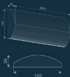
Молдинг LE-7
