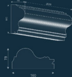
Карниз GE-11
