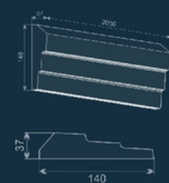
Молдинг LE-10
