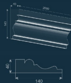
Молдинг LE-30
