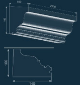
Карниз GE-12
