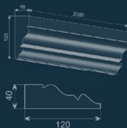
Молдинг LE-29A
