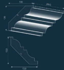
Фацет FE-12
