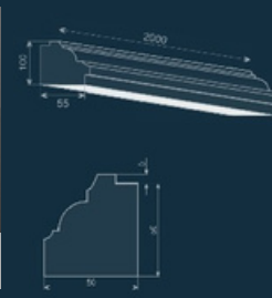
Рустова смуга LB-1A
