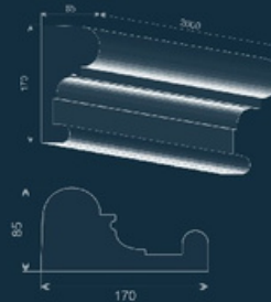
Карниз GE-14
