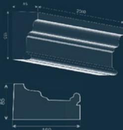
Карниз GE-16B
