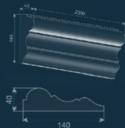
Молдинг LE-31
