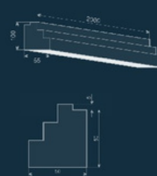
Рустова смуга LB-3A
