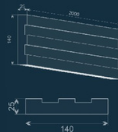
Молдинг LE-8
