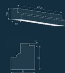
Рустова смуга LB-5A
