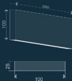
Молдинг LE-32
