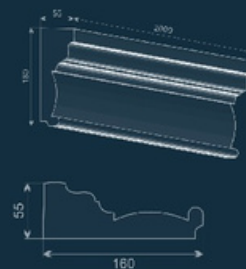
Карниз GE-10A
