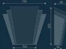
Замковий камінь ZE-5
