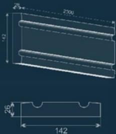
Молдинг LE-9
