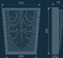
Замковий камінь ZE-2A
