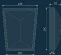
Замковий камінь ZE-1
