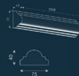
Молдинг LE-22
