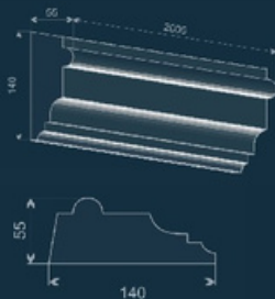
Молдинг LE-19
