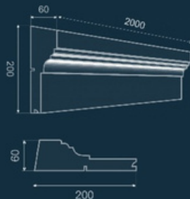
Карниз GE-4C
