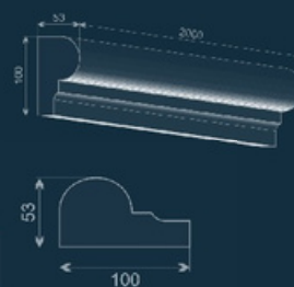
Молдинг LE-24
